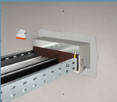
Potentialausgleich anschließen und Kennzeichnungsschild anbringen
